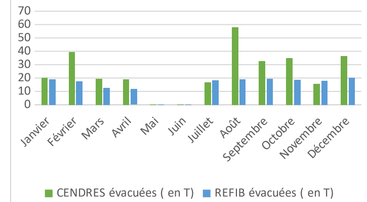
Evacuation cendres et refib - 2020
