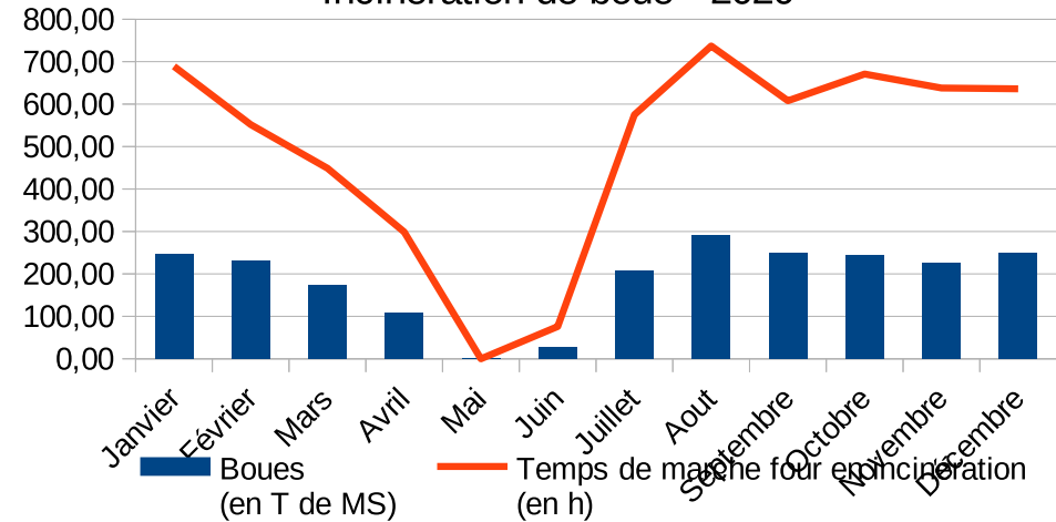
Incinération de boue - 2020
