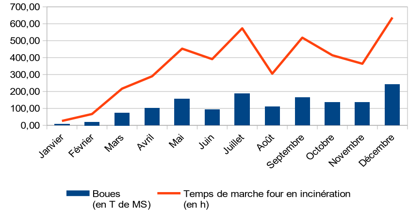
Incinération de boue - 2019
