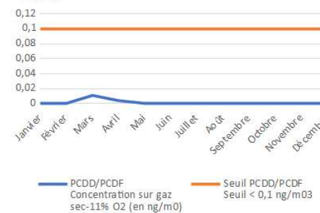
Suivi dioxines/furanes en sortie de cheminée - 2020
